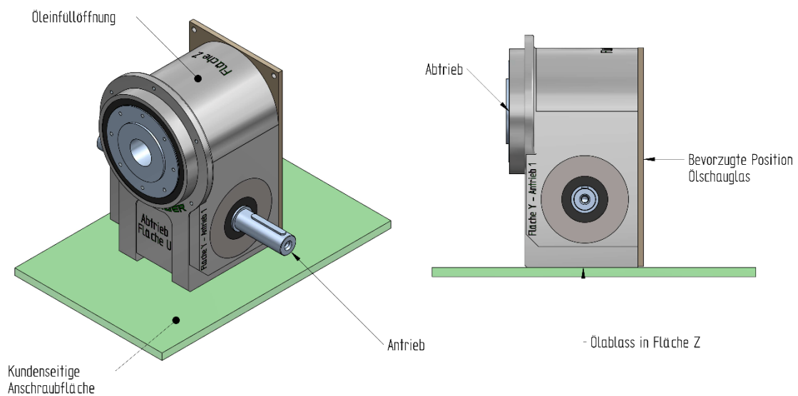
Abbildung 5: Einbaulage D
