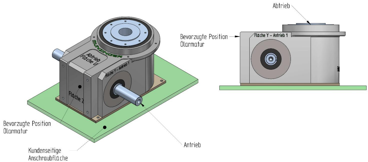
Abbildung 4: Einbaulage B
