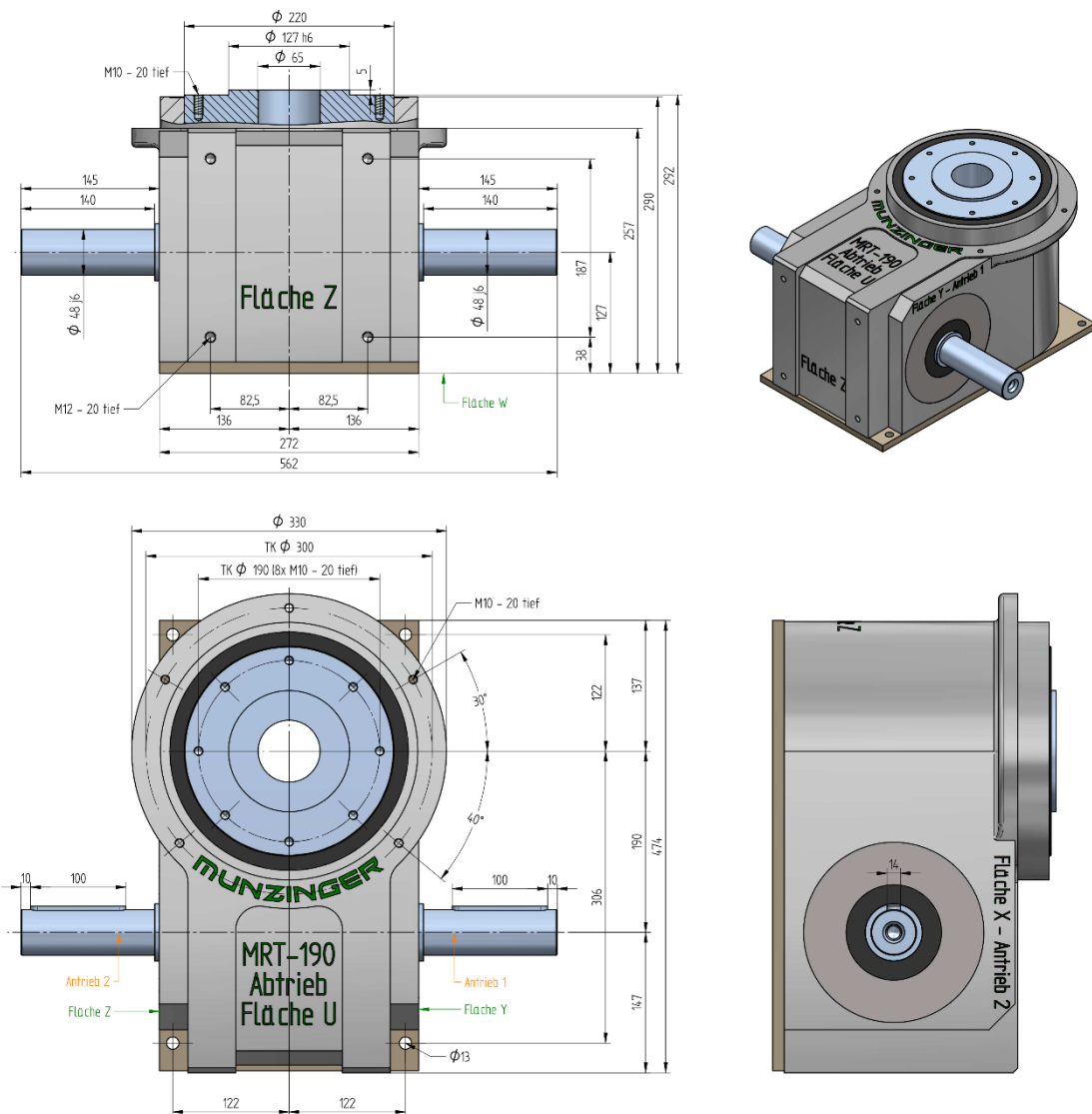
Abbildung 3: Abmessungen der Getriebe
